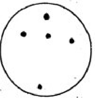
Cygnus
