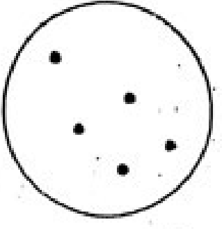
Cepheus
