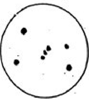
Orion
