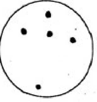
Cygnus
