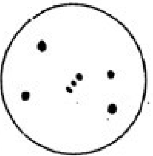
Orion
