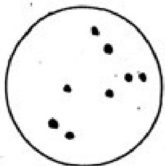
Gemini
