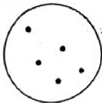
Cepheus
