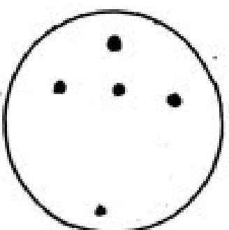
Cygnus
